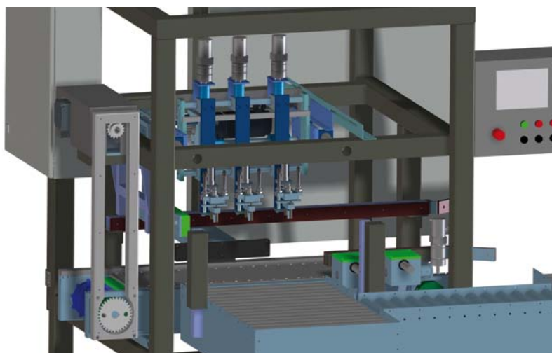
Mit Hilfe von Messtastern wird die Stopfenhöhe in Relation zur Deckeloberfläche geprüft.
